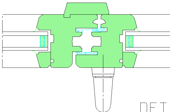
EN OPTION SUR CHASSIS STANDARD ET RUSTIQUE MAUCLAIR MOULURE DE 22 mm
